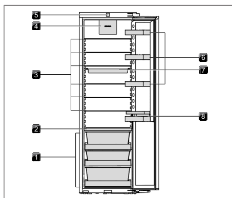
Abb. 5.1 Aufbau C178K
