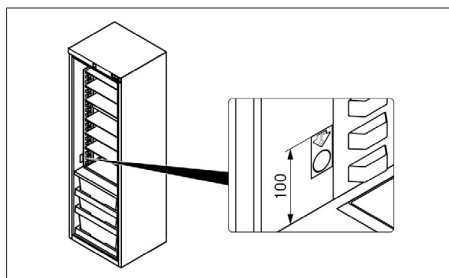
Abb. 8.16 Temperaturindikator platzieren
